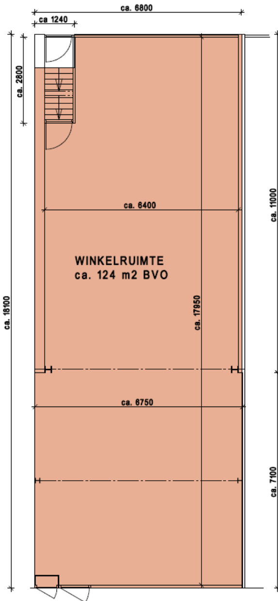
BEGANE GROND NIEUWE SITUATIE
